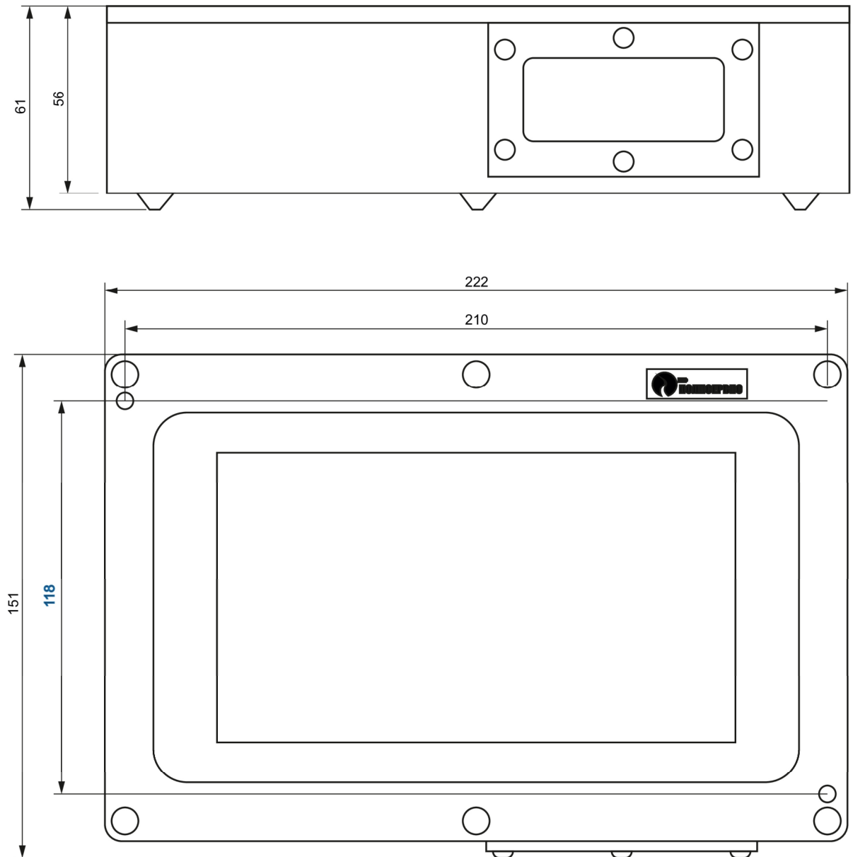
Рисунок 1 - Габаритный чертеж БОС-3-2-К
